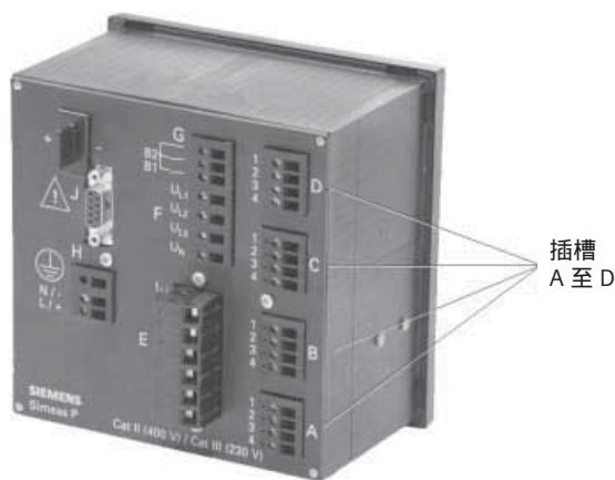
图 13/61 带输入和输出模块的 SIMEAS P610/P660
