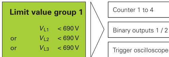
图 13/59 限值
