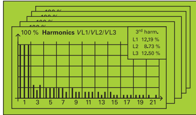
图 13/48 通过四个按钮最多可显示 20 个屏幕 (SIMEAS P610)
