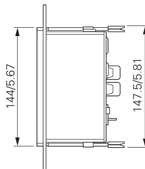
SIMEAS P650/660
