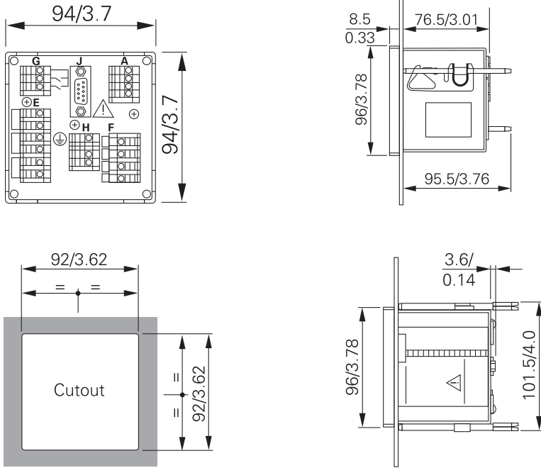
SIMEAS P50 图 16/41
