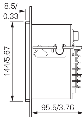
SIMEAS P650/P660
