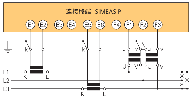
图 13/74 三线制三相
