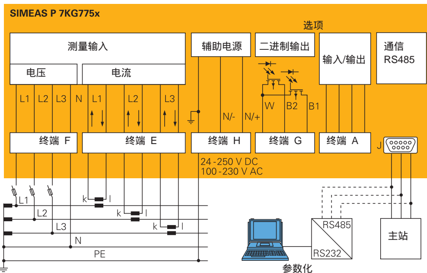
图 13/47 输入/输出
