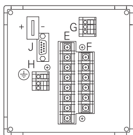
SIMEAS P650
