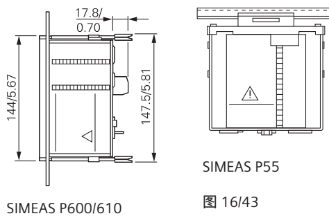
SIMEAS P600/P610
