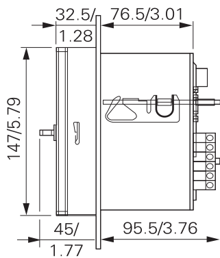
SIMEAS P6xx 带透明塑料面板, 面板保护等级为 IP54
